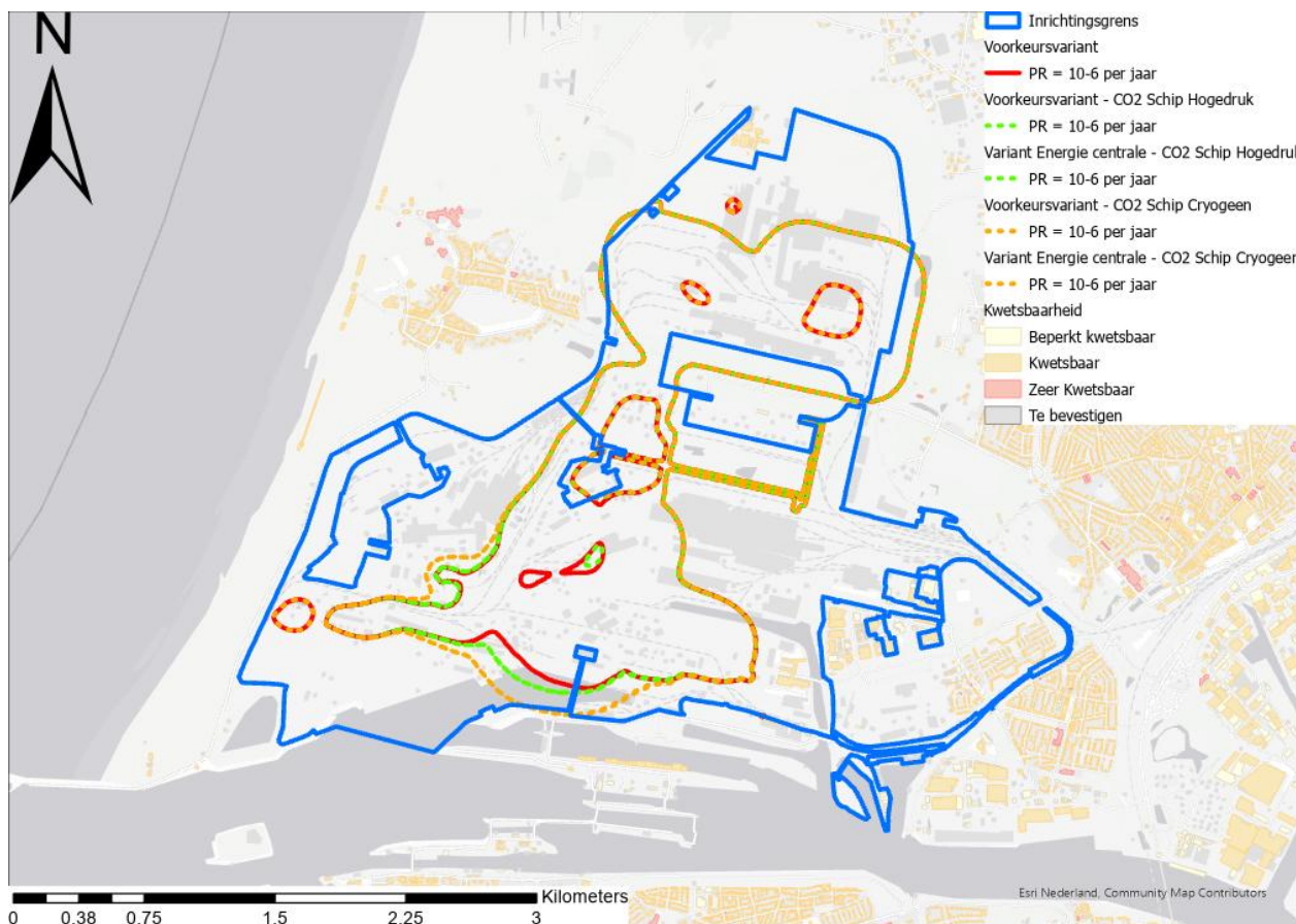
Figuur 12.6 Plaatsgebonden risicocontouren van 10 -6 per jaar voor elke variant waarbij CO 2 export per schip plaatsvindt. De contouren zijn verschillend georiënteerd in het gebied gemarkeerd door de zwarte cirkel; buiten dit gebied vallen de contouren exact op elkaar waar door deze moeilijk te onderscheiden zijn in de afbeelding.
