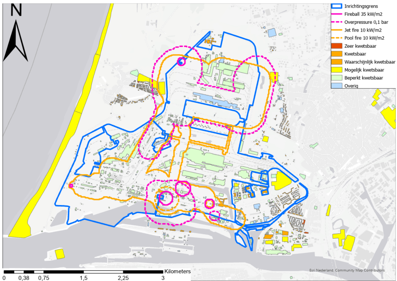
Figuur 12.7 Explosie- en brandaandachtsgebieden in de referentiesituatie
